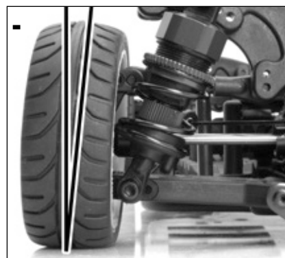
- negativer Sturz negative Camber Carrossage négatif Camber negativo
