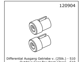
120904 Differential Ausgang Getriebe v. (2Stk.) - S10 Outdrive Gear Box front (2pcs) - S10
